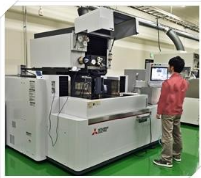
ワイヤ放電加工機
